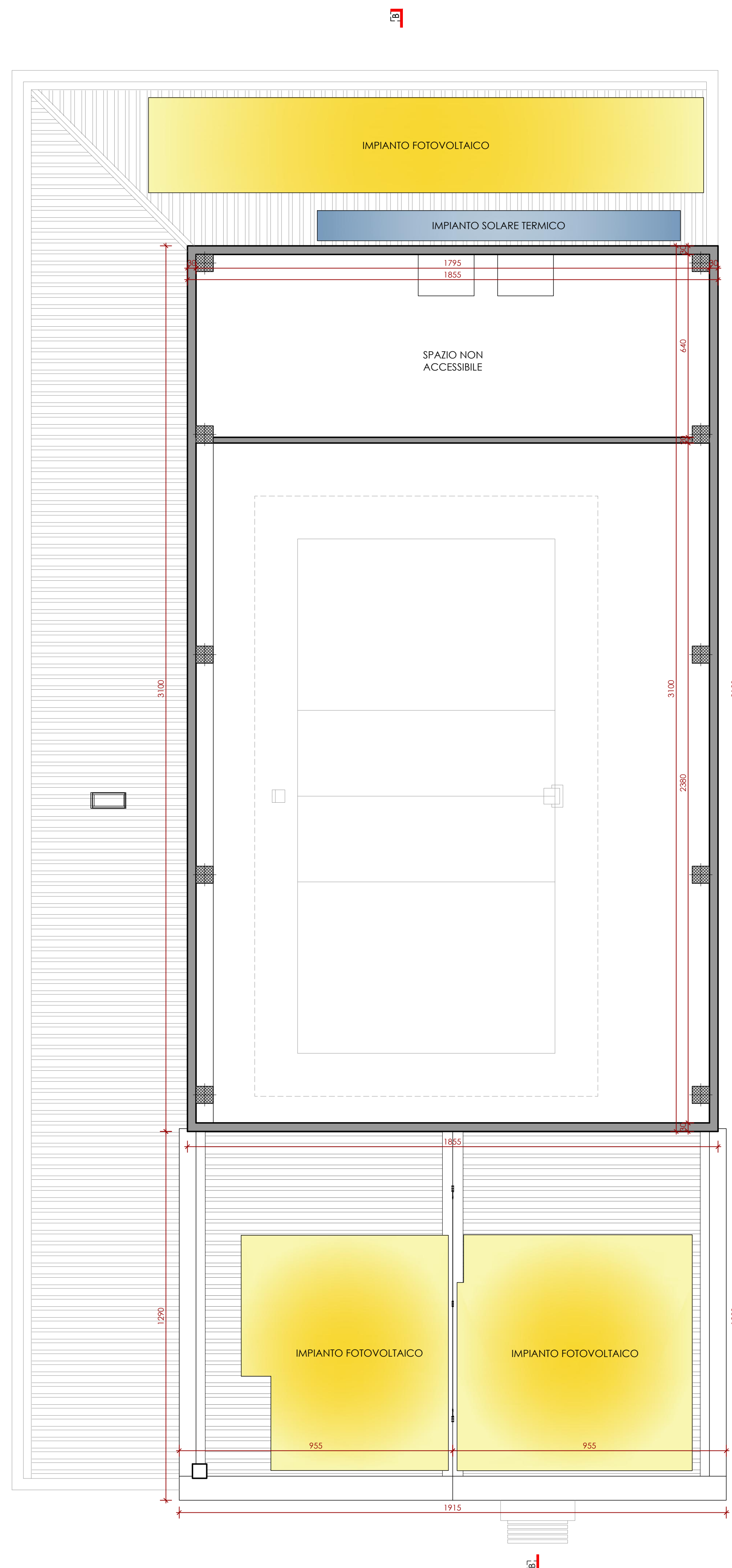
Pianta a QUOTA +7,00m
